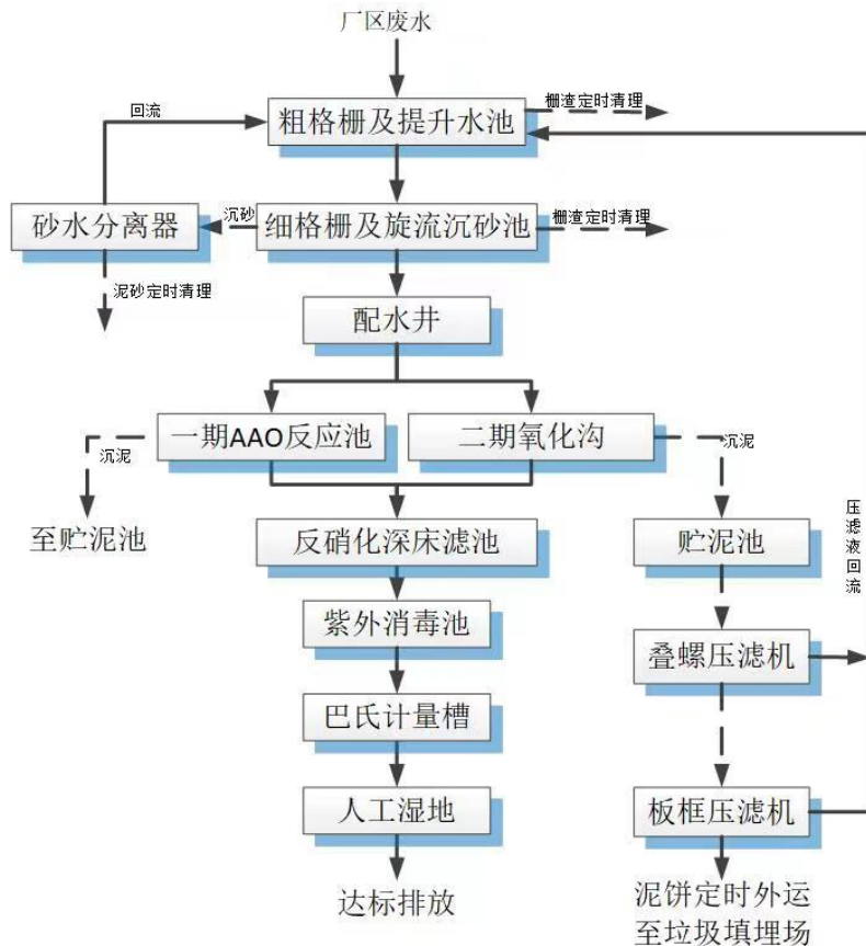
西海镇污水处理厂工艺流程框图
